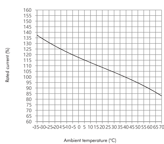
NXMLE-160(W125) 25A-63A
