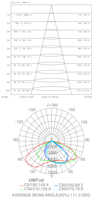
LUMAX 150W NEMA 3
