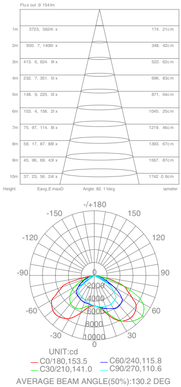
LUMAX 200W NEMA 3
